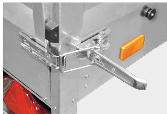
Preklopni zatvarači na stražnjoj stranici
