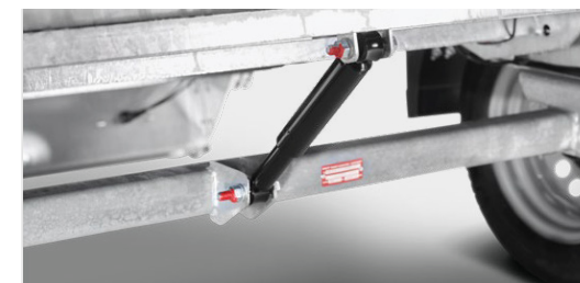
Nagibni sanduk (kod HA nagibne izvedbe) s amortizerom za nagibnu funkciju
